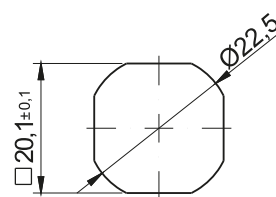
Монтажное отверстие
