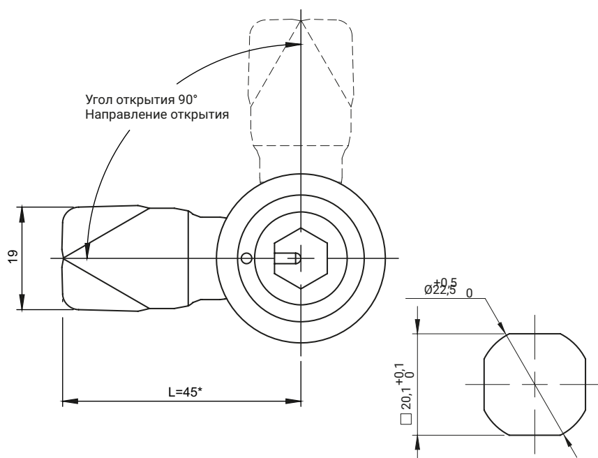
Монтажное отверстие
