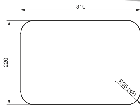
Монтажные отверстия
