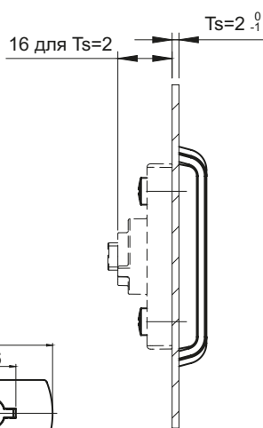
RW120.N (замок под накладку)
