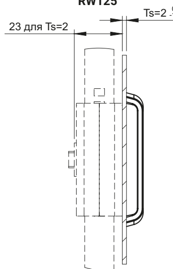
RW120.M (замок под зубчатый механизм)
